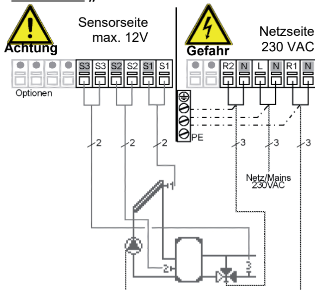
Abb. 3.2.5 „Solar mit Rücklaufanheb.“
