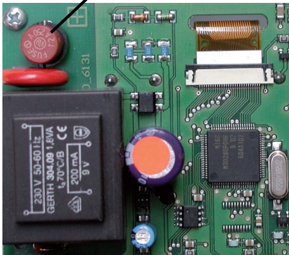
Abb. 3.1.1 Sicherung
