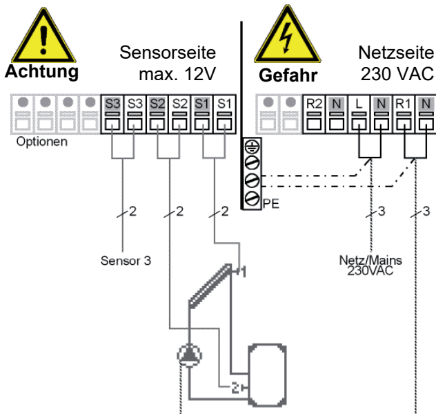
Abb. 3.2.2 „Solar mit Speicher“
