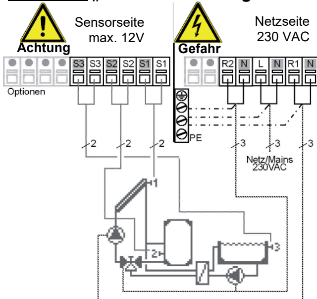
Abb. 3.2.14 „Universal 2x \Delta T -Regler“
