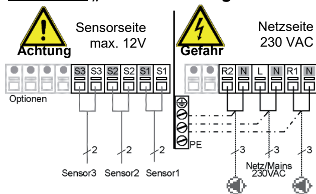
Abb. 3.2.13 „Universal ΔT-Regler“
