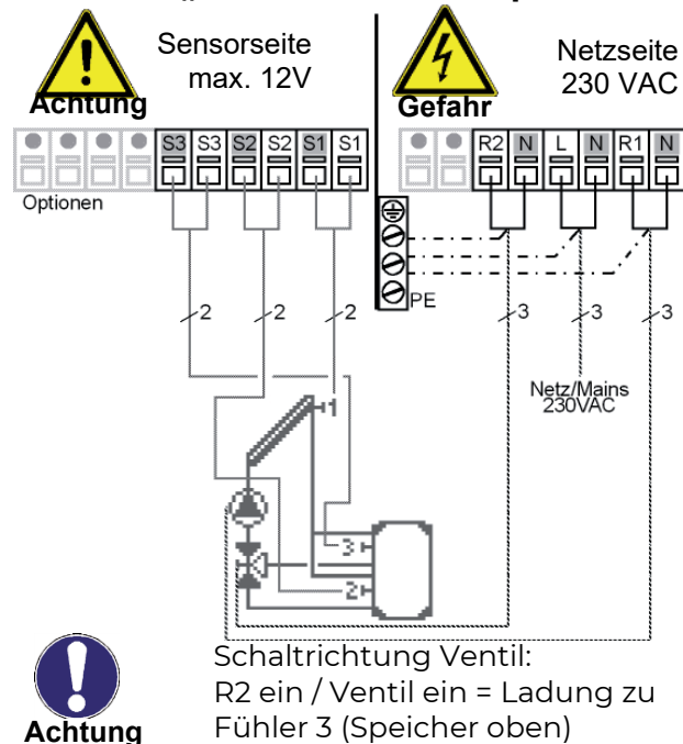
Abb. 3.2.6 „Solar mit 2 Zonenspeicher“
