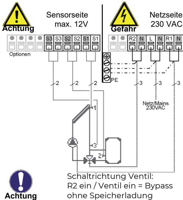
Abb. 3.2.4 „Solar mit Bypass“
