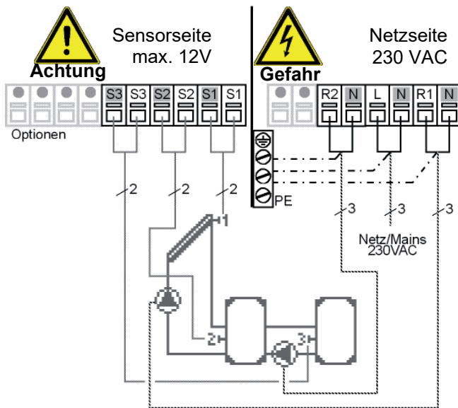
Abb. 3.2.12 „Solar mit Folgespeicher“
