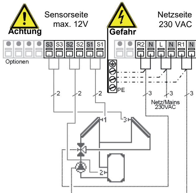
Abb. 3.2.8 „Solar 2 Koll. (Ost/West)“
