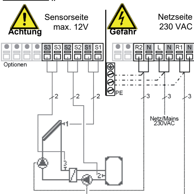
Abb. 3.2.7 „Solar mit ext. W-Tauscher“
