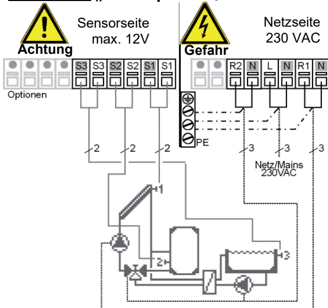
Abb. 3.2.14 „Solar Speicher/Pool“
