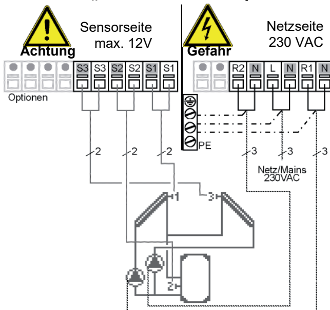
Abb. 3.2.9 „Solar 2 Koll. 2 Pumpen“
