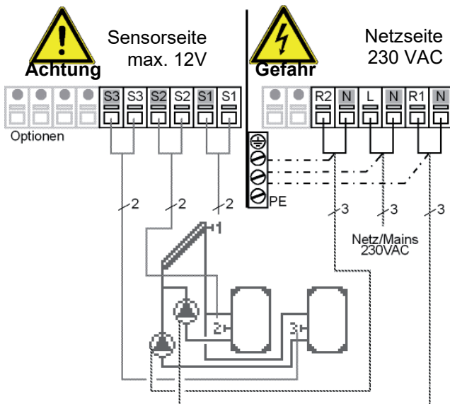
Abb. 3.2.11 „Solar 2 Speicher/2 Pu.“
