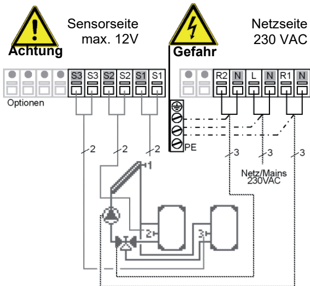
Abb. 3.2.10 „Solar 2 Speicher/Ventil“
