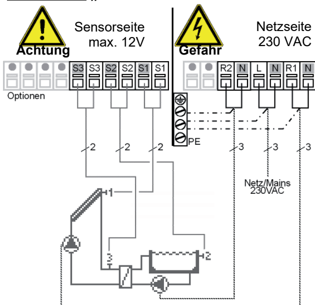
Abb. 3.2.13 „Solar mit Schwimmbad“
