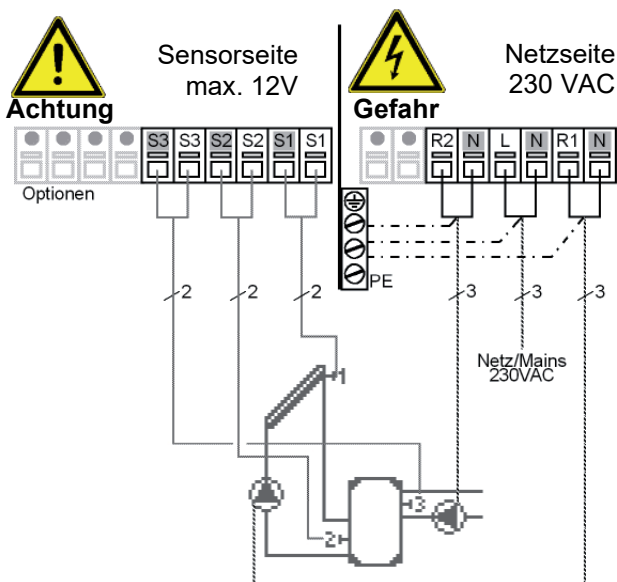
Abb. 3.2.3 „Solar + Thermostat“
